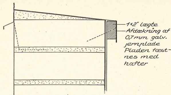
Fig. 8. Afdækning af murkam med metalplade.
