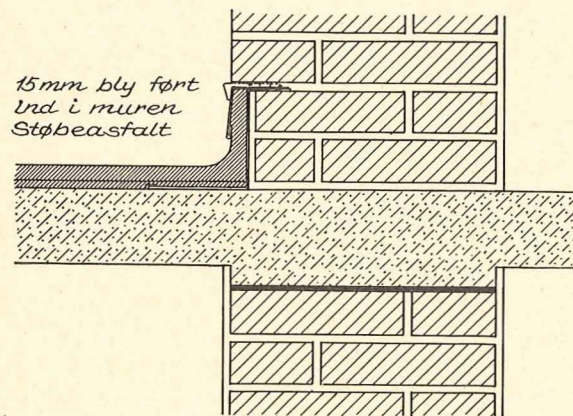
Fig. 12. Inddækning med zinkindskud og blyplade mellem mur og betontag med asfalt.
