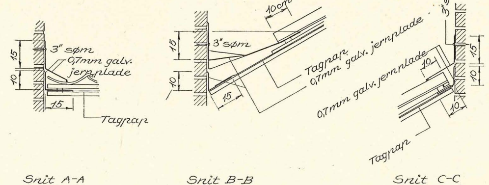
Fig. 10. Inddækninger mellem skorsten og tegltag som de almindeligt udføres i Sverige.
