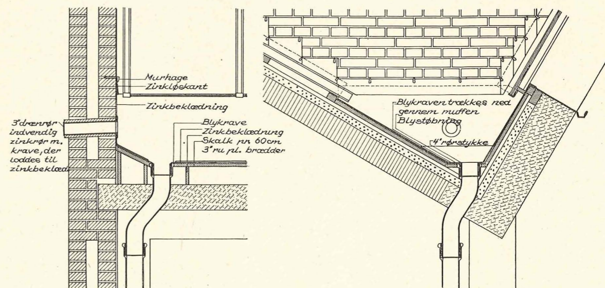
Fig. 23. Skotrende ved shedtag med ovenlys.
