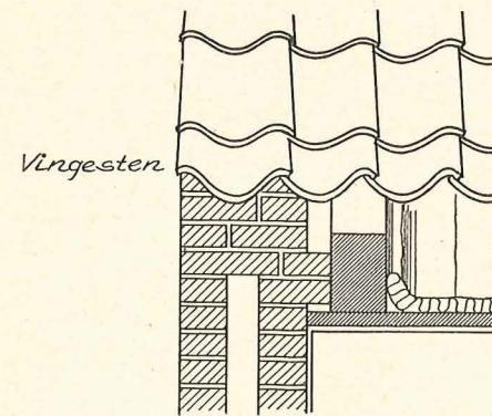
Fig. 9. Gavl inddækket med dobbeltfalsede tagsten.
