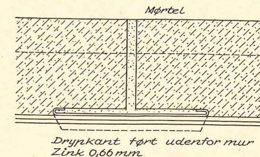
Fig. 4. Stødfuge mellem betonafdækningssten med indlagt metalplade.
