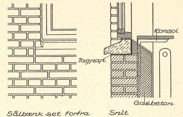
Fig. 18. Betonsålbænk, ført et stykke ind i muren.
