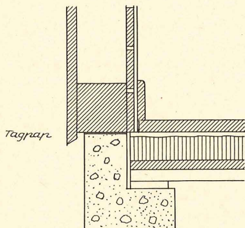
Fig. 25. Betonfundament ved træhus tilbagetrukket fra facadelinjen, så regnvand løber af.
