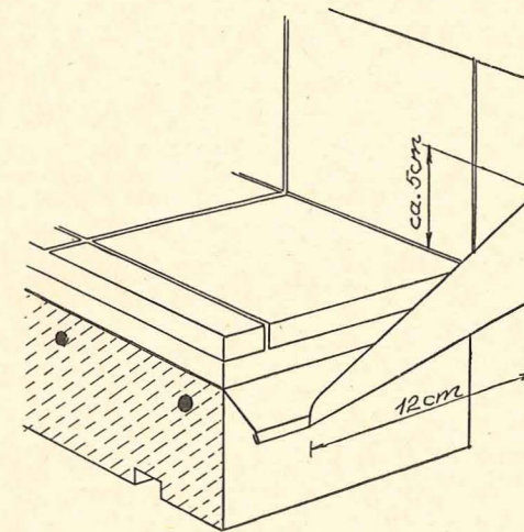
Fig. 16. Vandudleder ved altanplades tilslutning til mur.
