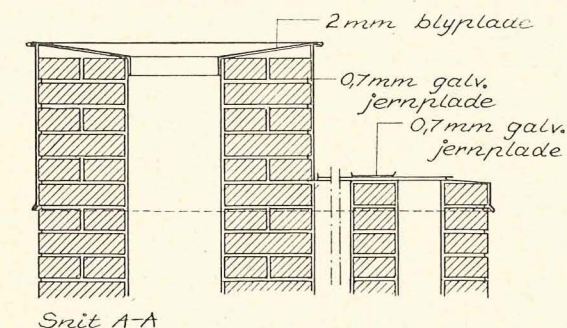
Snit A-A
