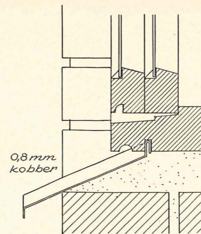
Fig. 22. Metalsålbænk ved trævindue.
