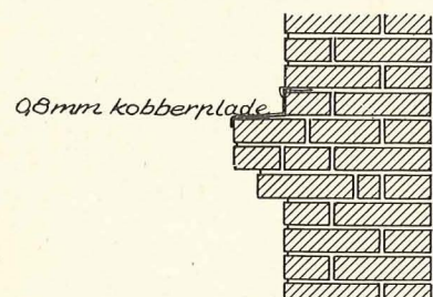
Fig. 7. Afdækning af gesimsliste med metalplade.
