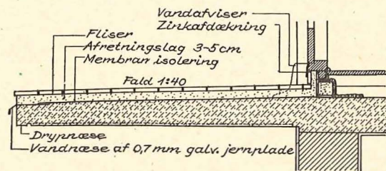
Fig. 15. Altanplade, isoleret mod fugtgennemtrængning.
