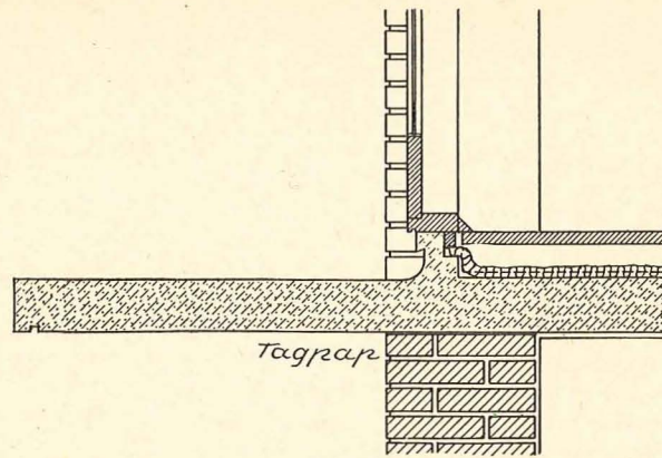
Fig. 14. Altanplade med forhøjelse til dørtærskel.
