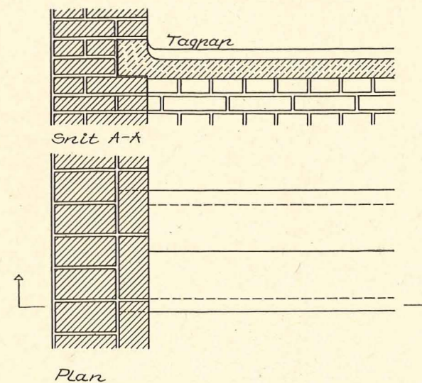
Fig. 17. Afdækningssten, ført 1/2 sten ind i tilstødende mur.
