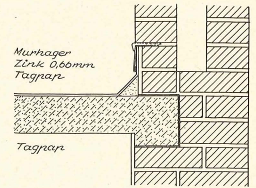
Fig. 11. Inddækning med zinkinds kud mellem mur og betontag med pap.
