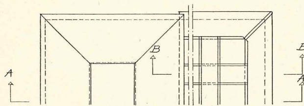
Fig. 6. Skorstensafdækning med blyplade, som den almindeligt udføres i Sverige.
