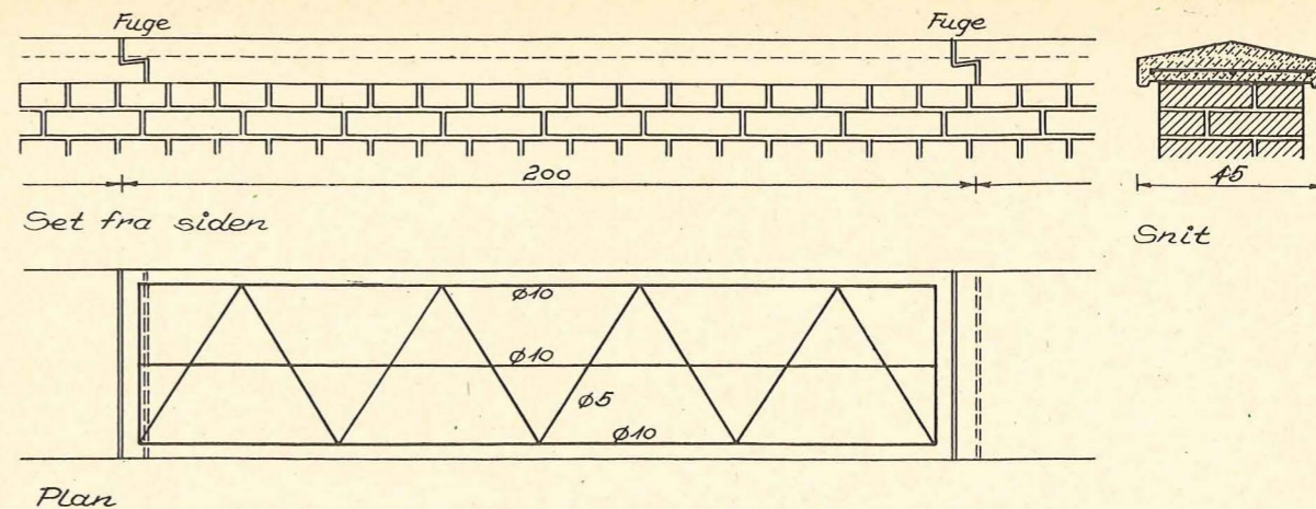
Fig. 3. Betonafdækningssten.
