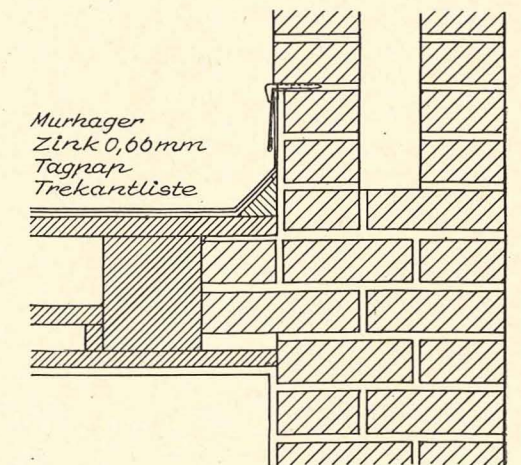
Fig. 19. Inddækning med zinkindskud mellem mur og trætag med tagpap.
